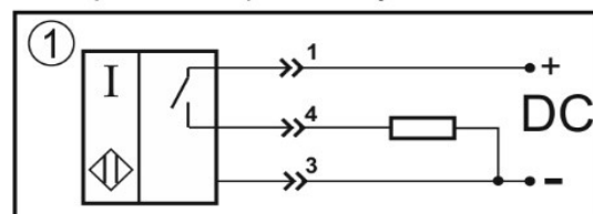
Нормально-разомкнутый контакт
