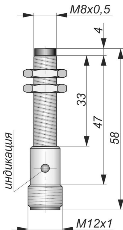
Габаритный чертеж
