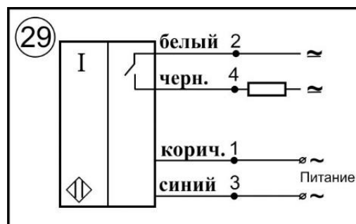
Схема соединения
