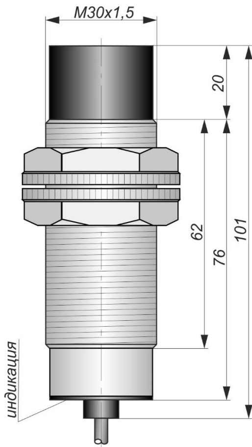
Габаритный чертеж
