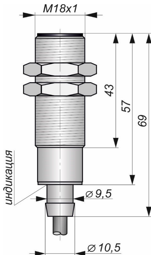
Габаритный чертеж
