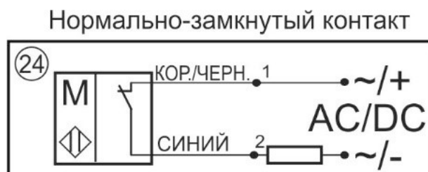
Схема соединения
