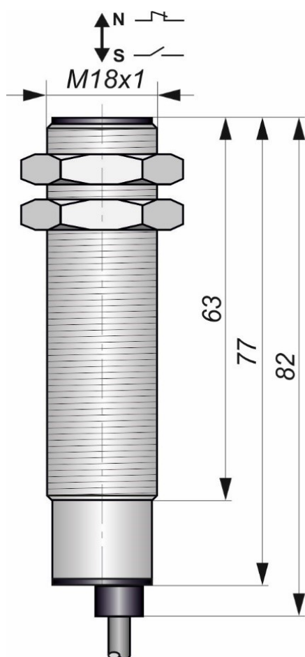
Габаритный чертеж
