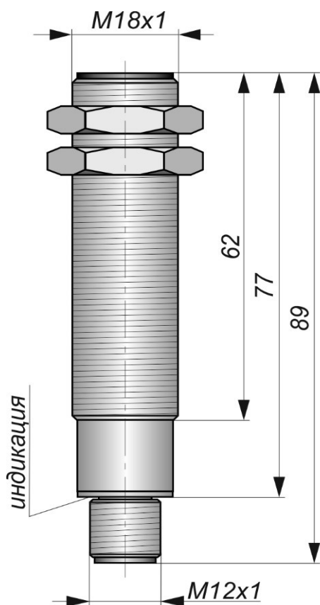
Габаритный чертеж
