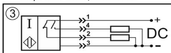
Переключающий контакт
