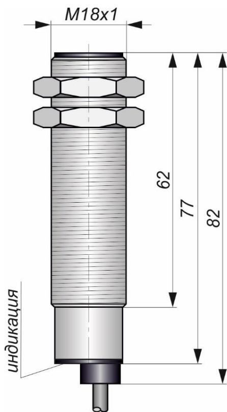
Габаритный чертеж
