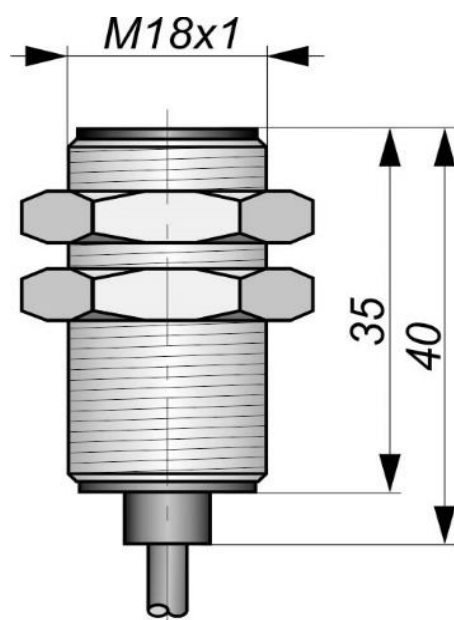
Габаритный чертеж
