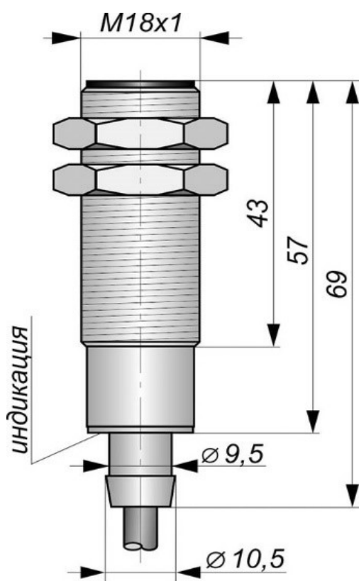
Габаритный чертеж
