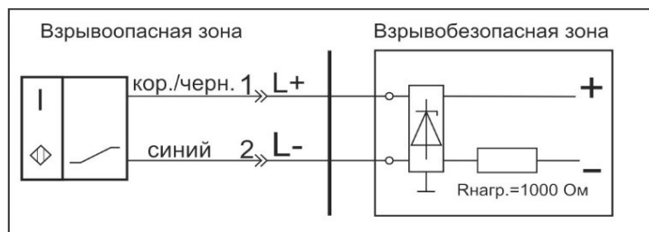
Схема соединения
