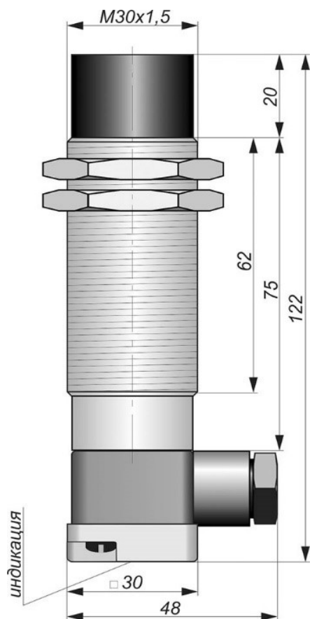
Габаритный чертеж
