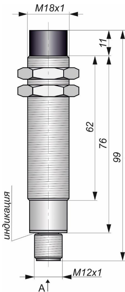
Габаритный чертеж
