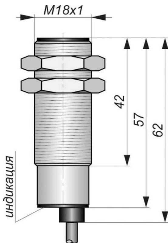
Габаритный чертеж
