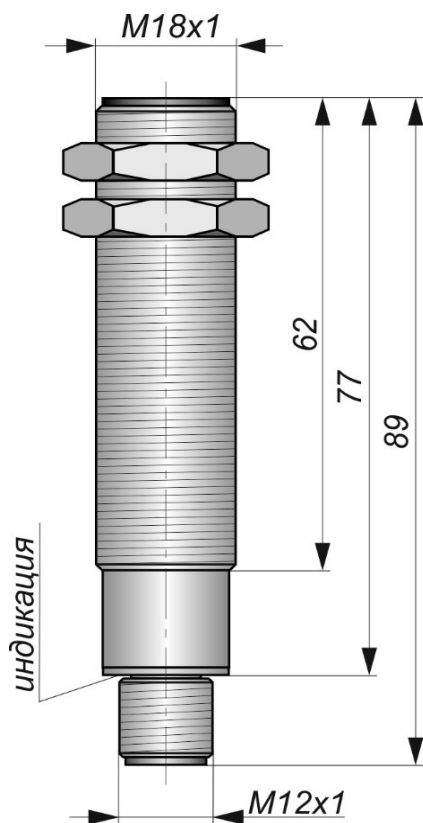
Габаритный чертеж
