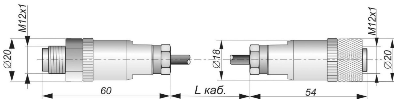
Габаритный чертеж
