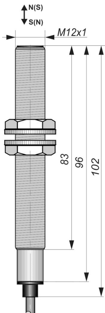
Габаритный чертеж
