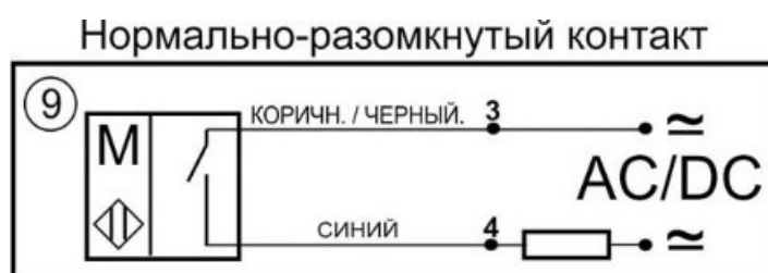
Схема соединения
