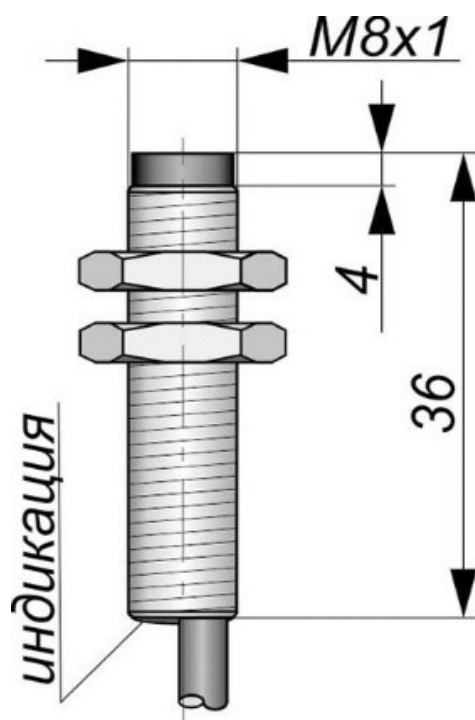
Габаритный чертеж
