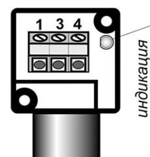
Цоколевка клеммной колодки
