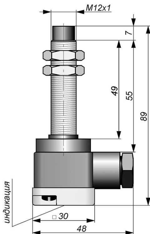
Габаритный чертеж
