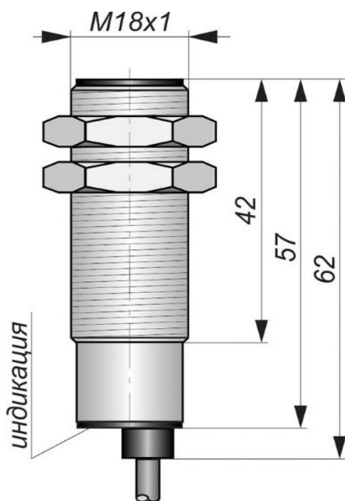
Габаритный чертеж
