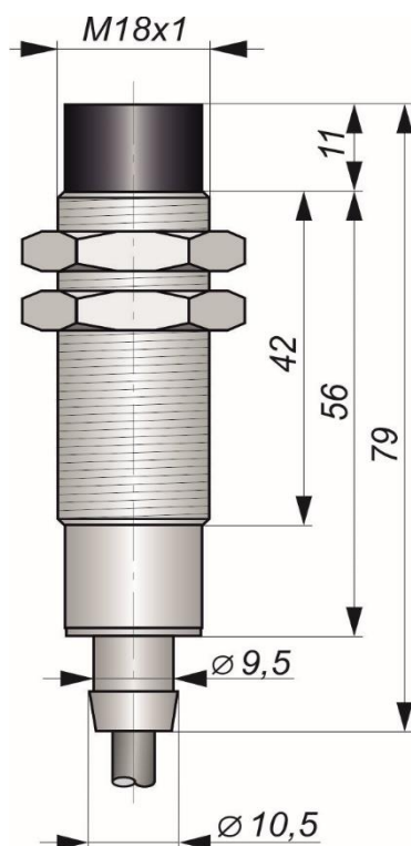
Габаритный чертеж
