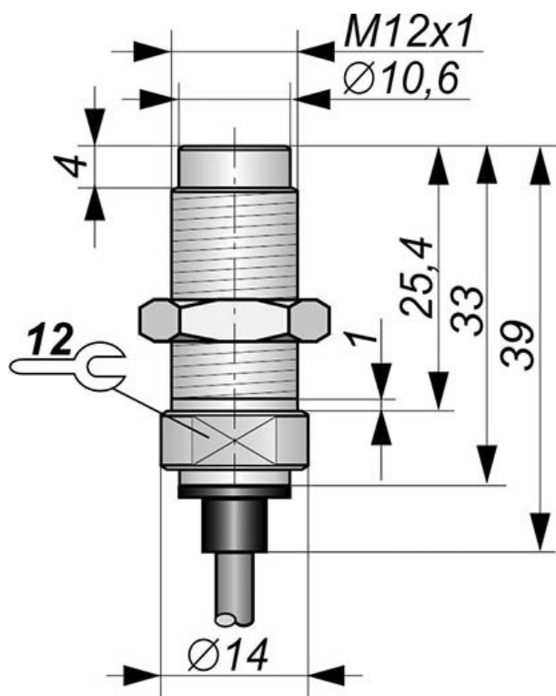
Габаритный чертеж
