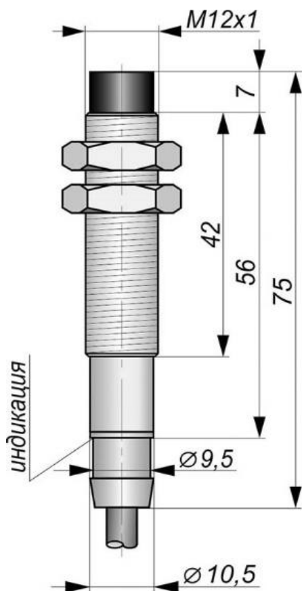
Габаритный чертеж
