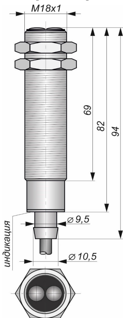
Габаритный чертеж
