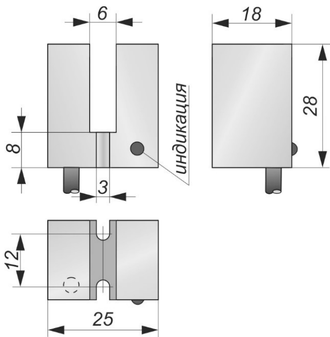
Габаритный чертеж
