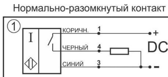
Схема соединения
