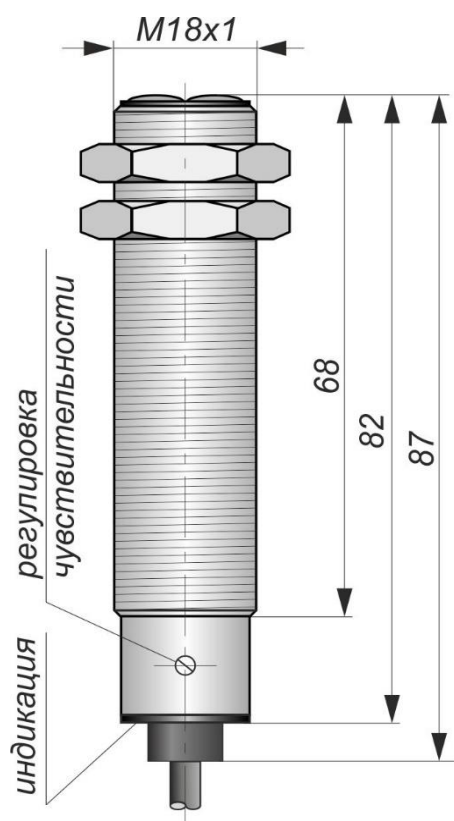
Габаритный чертеж
