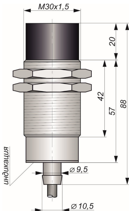
Габаритный чертеж
