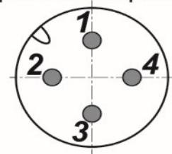
Цоколевка разъема
