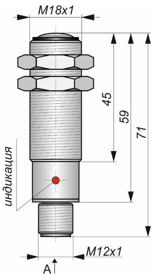
Габаритный чертеж
