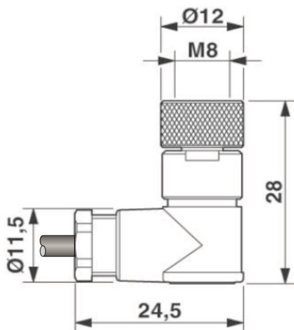
Габаритный чертеж
