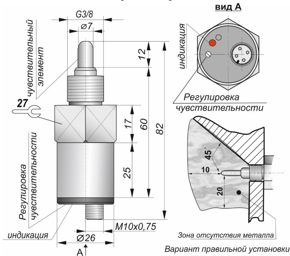
Габаритный чертеж
