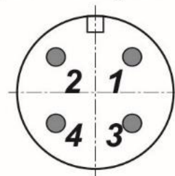
Цоколевка разъема
