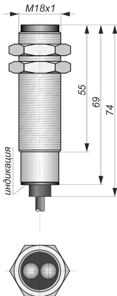
Габаритный чертеж
