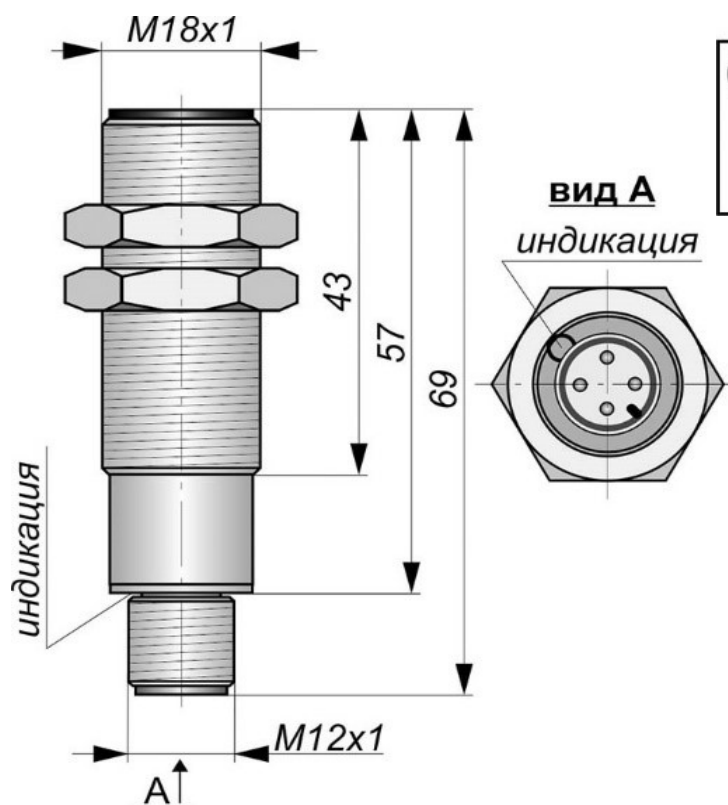
Габаритный чертеж
