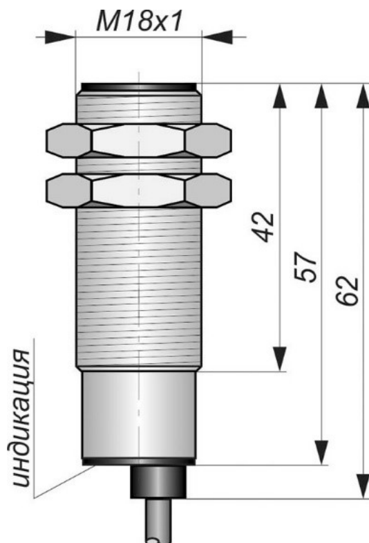
Габаритный чертеж
