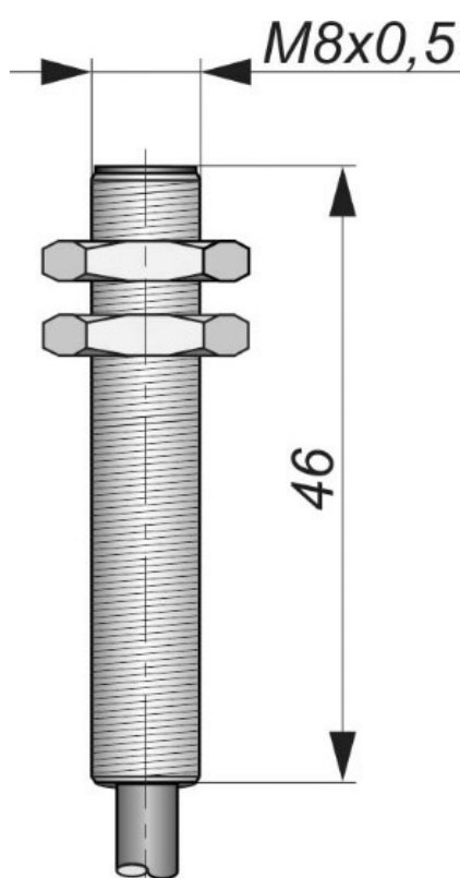
Габаритный чертеж
