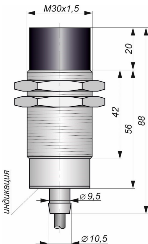
Габаритный чертеж
