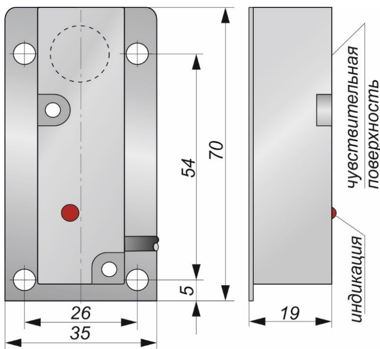
Габаритный чертеж
