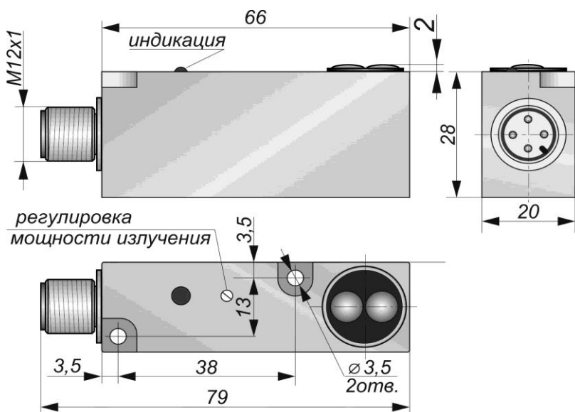
Габаритный чертеж
