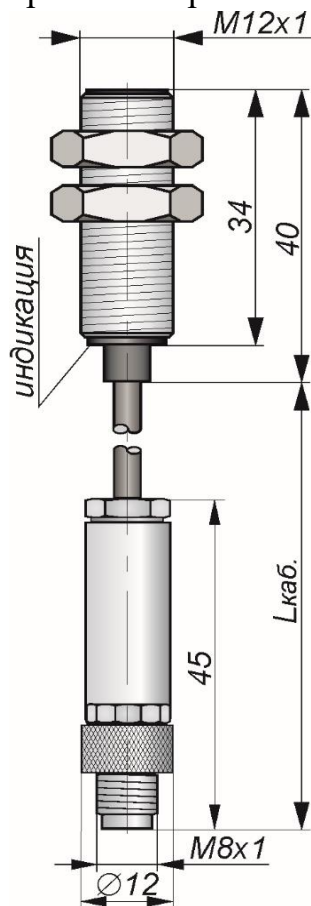
Габаритный чертеж
