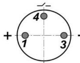
Цоколевка разъема
