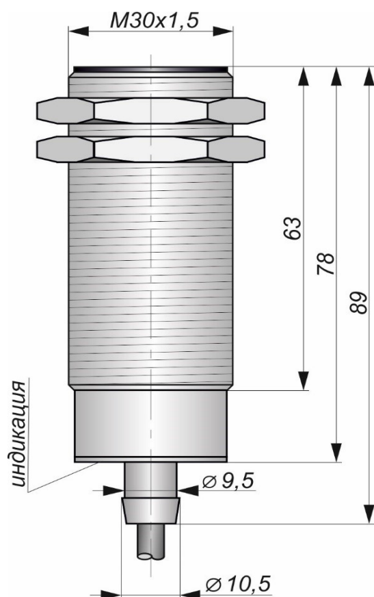
Габаритный чертеж
