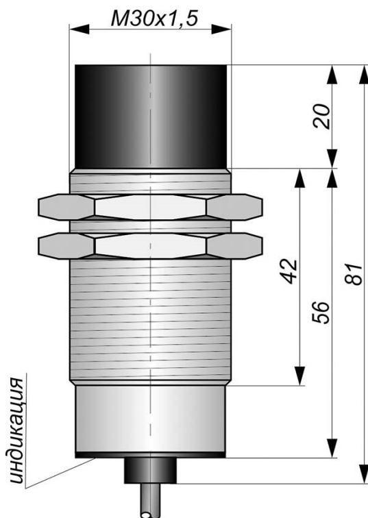
Габаритный чертеж
