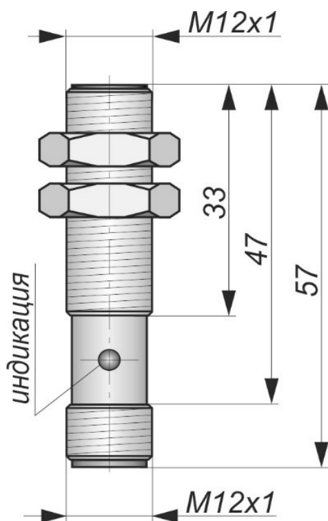
Габаритный чертеж
