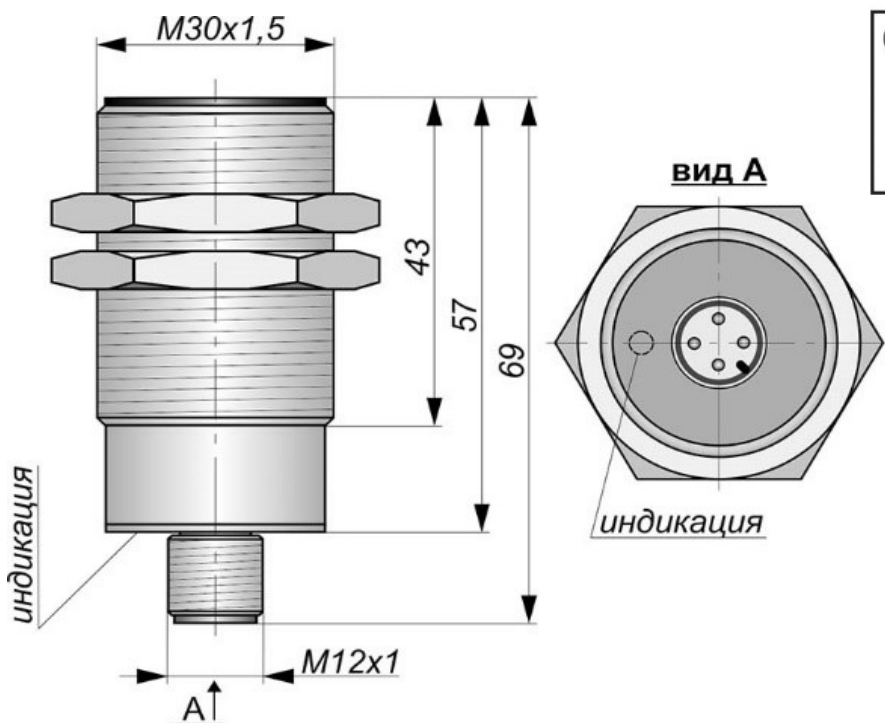
Габаритный чертеж
