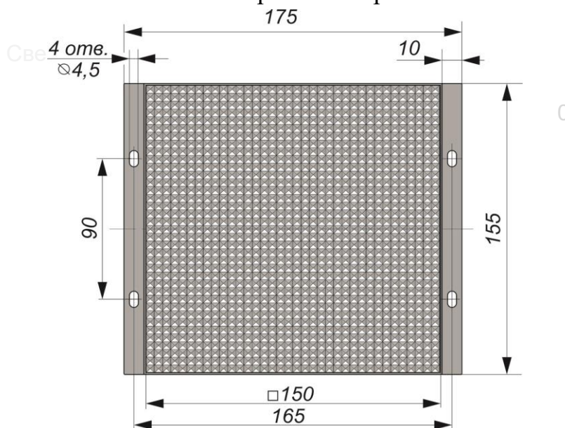
Габаритный чертеж
