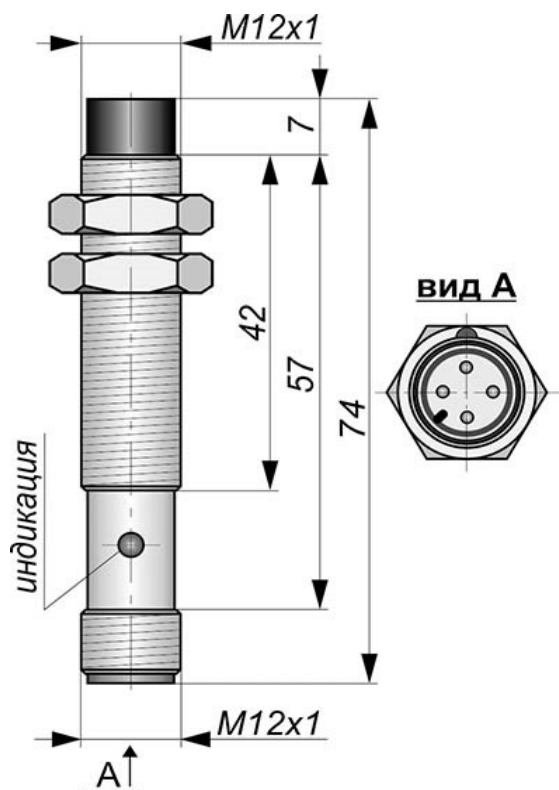
Габаритный чертеж
