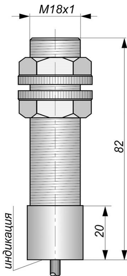
Габаритный чертеж
