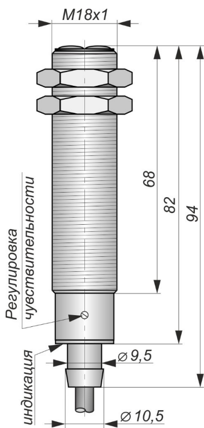
Габаритный чертеж
