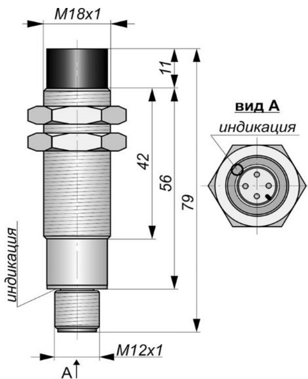
Габаритный чертеж
