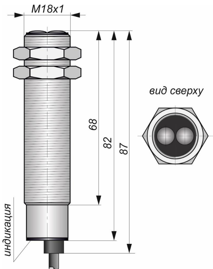
Габаритный чертеж
