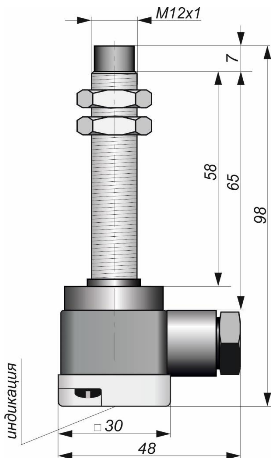
Габаритный чертеж
