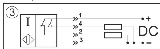
Переключающий контакт
