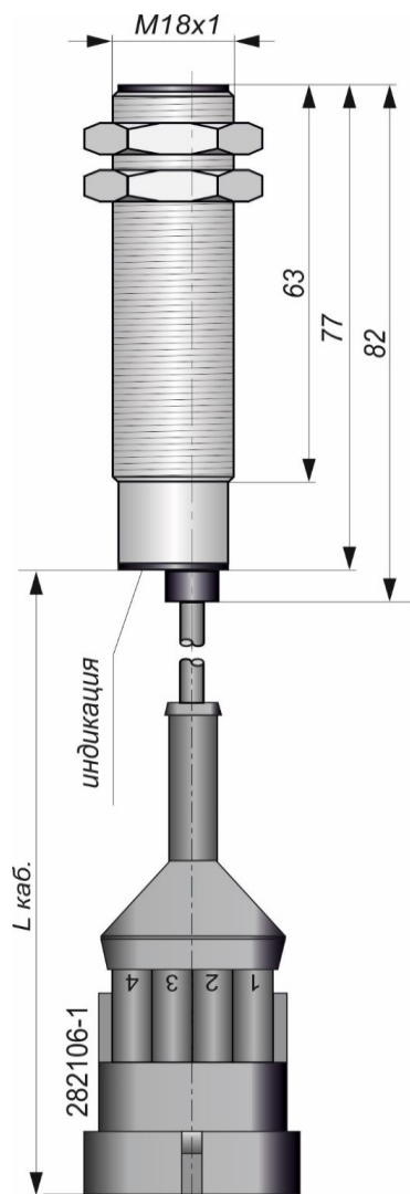
Габаритный чертеж
