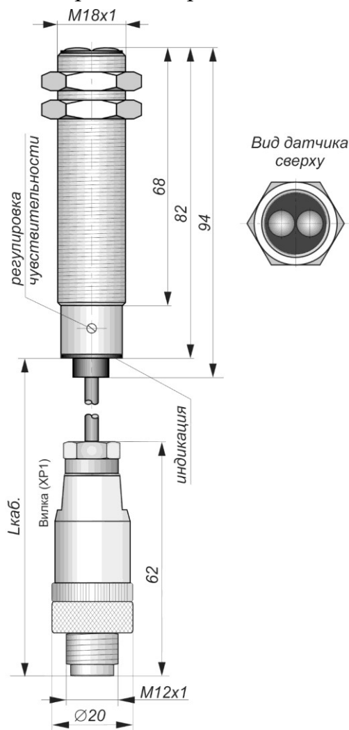
Габаритный чертеж
